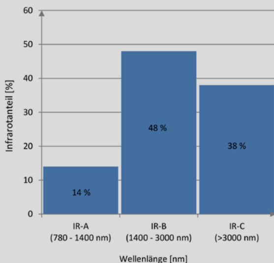
Infrarotspektrum der Sunlight-Infrarotstrahler
