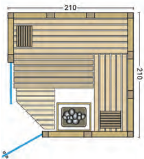
Abbildung Classico Fichte mit Sonderausstattung: EckEinstieg mit Tür ohne Schwelle, großes Glaselement, LED-Beleuchtung, Verdampferofen, Steuerung Saunacontrol C0.
